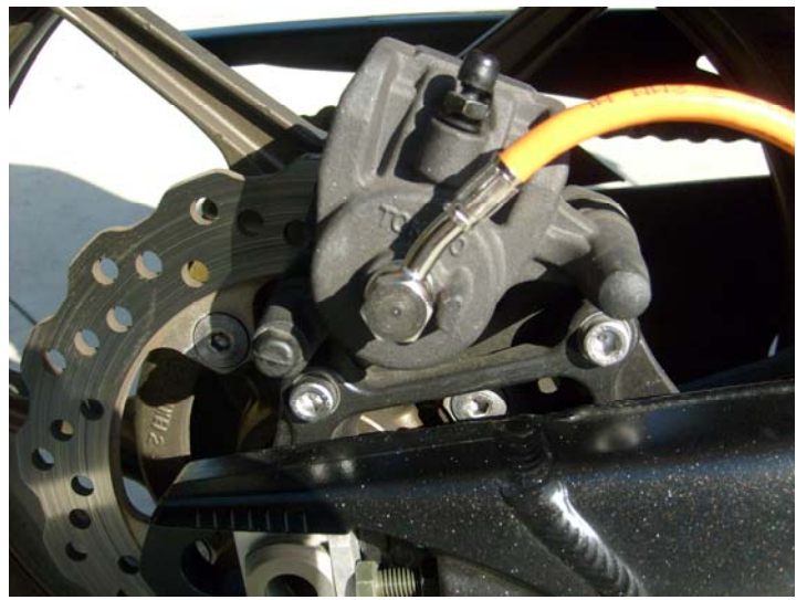
b. Rear caliper
